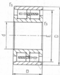
双列圆柱滚子轴承 NN型
