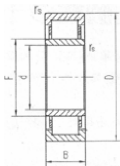
单列圆柱滚子轴承 NU型
