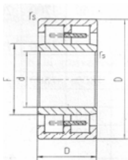
双列圆柱滚子轴承 NNU型
